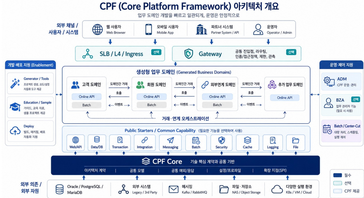
그림 1. CPF 전체 아키텍처 및 기능 영역
